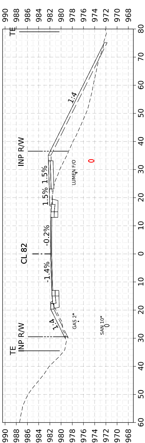
STA 114+50.00
